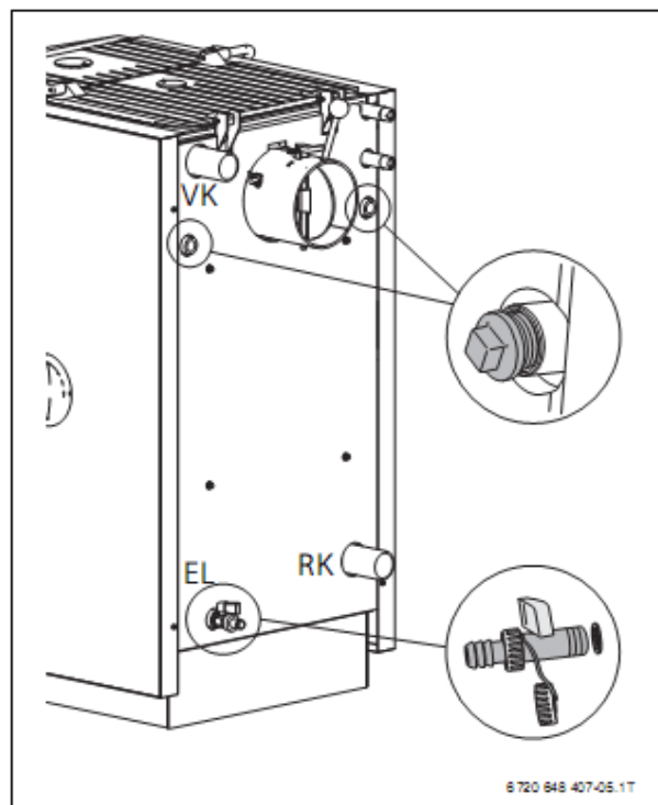
Obr. 11 Instalace hydraulických připojení
