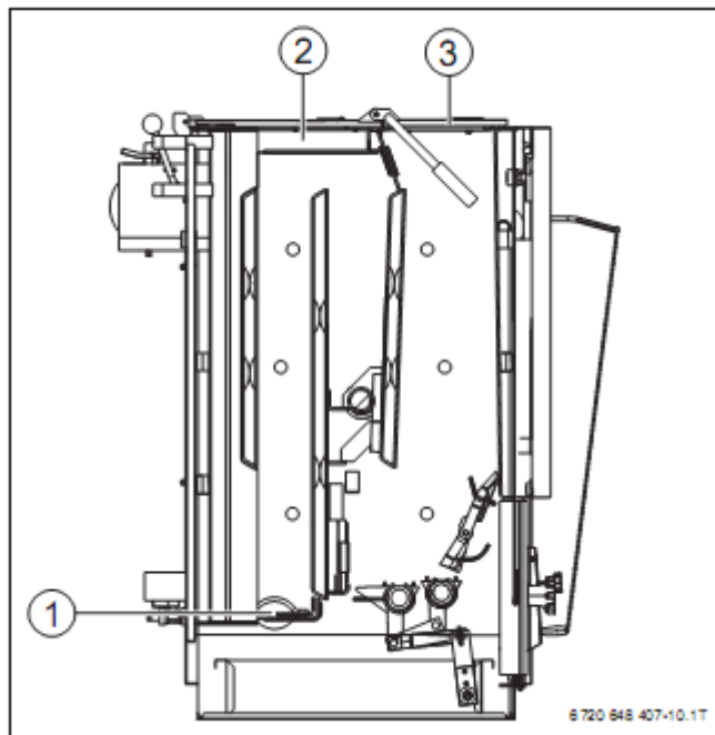
Obr. 39 Řez kotlem
