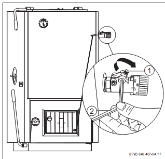
Obr. 7 Montáž regulátoru spalování
