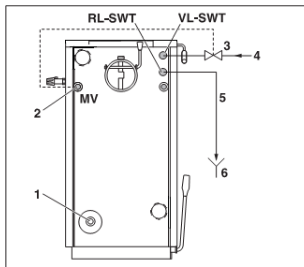
Obr. 12 Připojení bezpečnostního výměníku tepla
