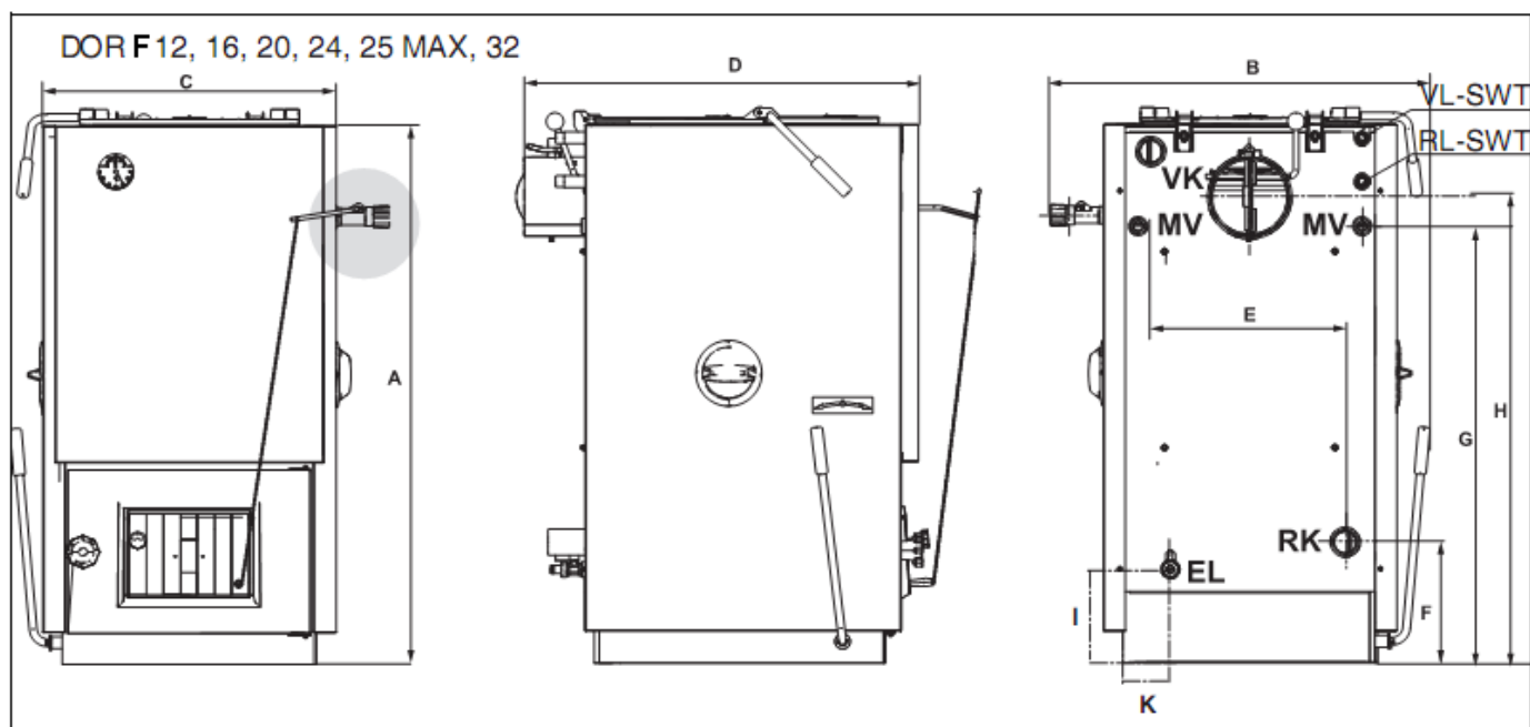
Obr. 3 Přípojky a rozměry
