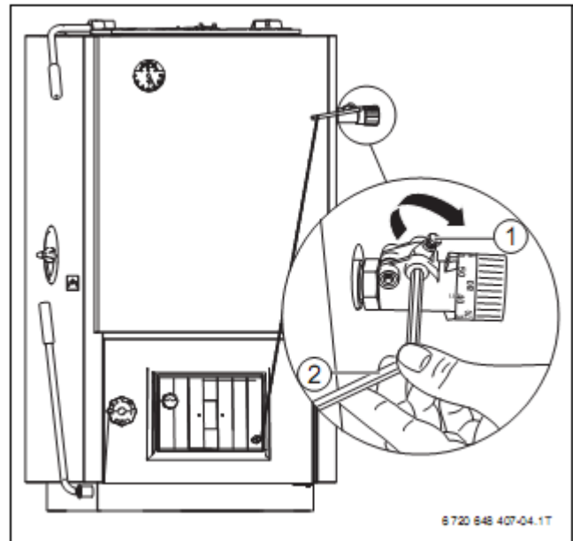
Obr. 20 Nastavení napětí řetězu
