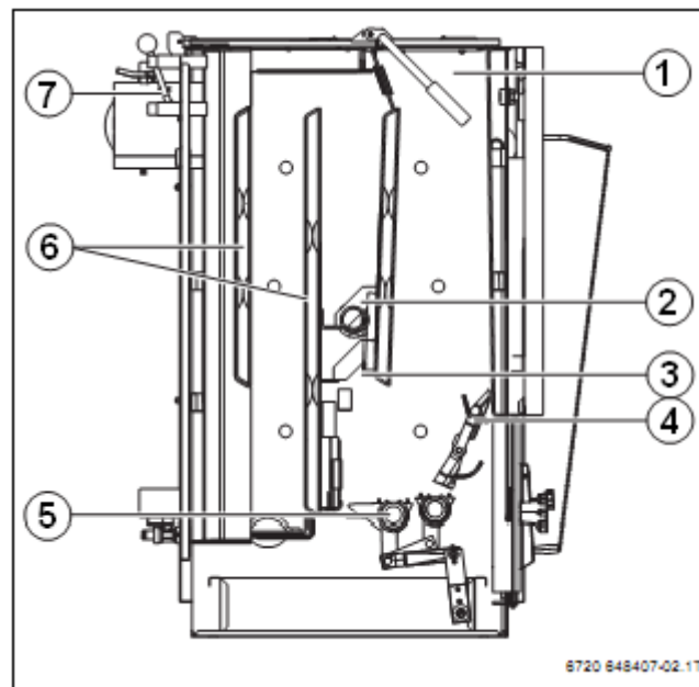
Obr. 2 Řez kotlem, zde např. typ 24
